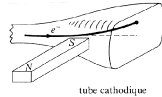
déviations d'un faisceau d'électrons par un aimant
